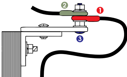
Figura 1 Ligação de terminais
